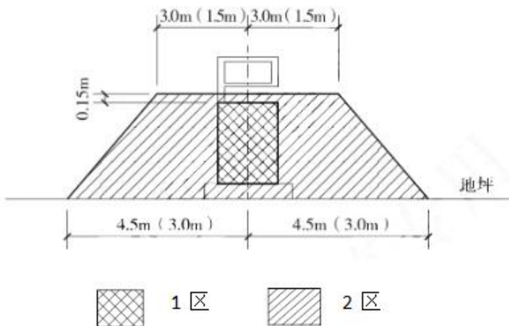
图3.12-2 汽油加油机爆炸危险区域划分
